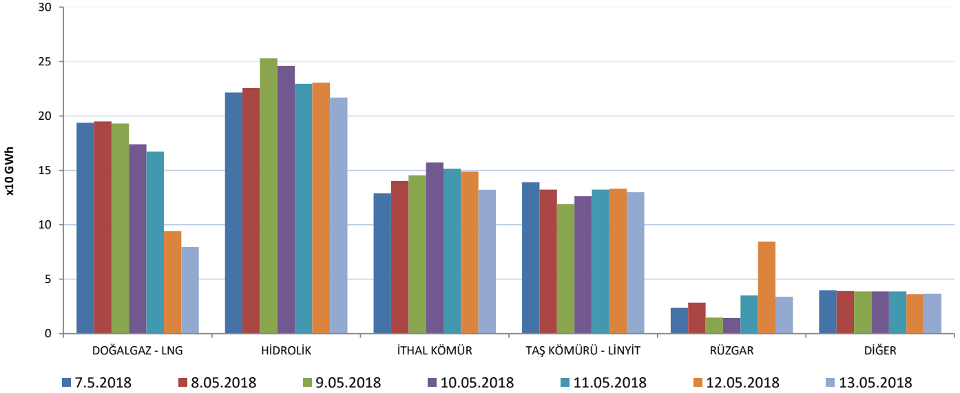
TÜRKİYE ELEKTRİK ÜRETİMİNİN BİRİNCİL KAYNAKLARA GÖRE DAĞILIMI
