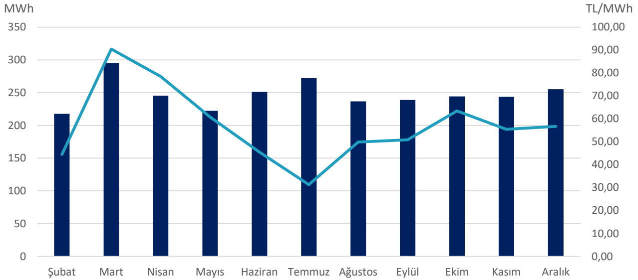
Grafik 40: Aylık Ortalama PFK Rezerv Miktarı ve Ağırlıklı Ortalama Fiyatı
