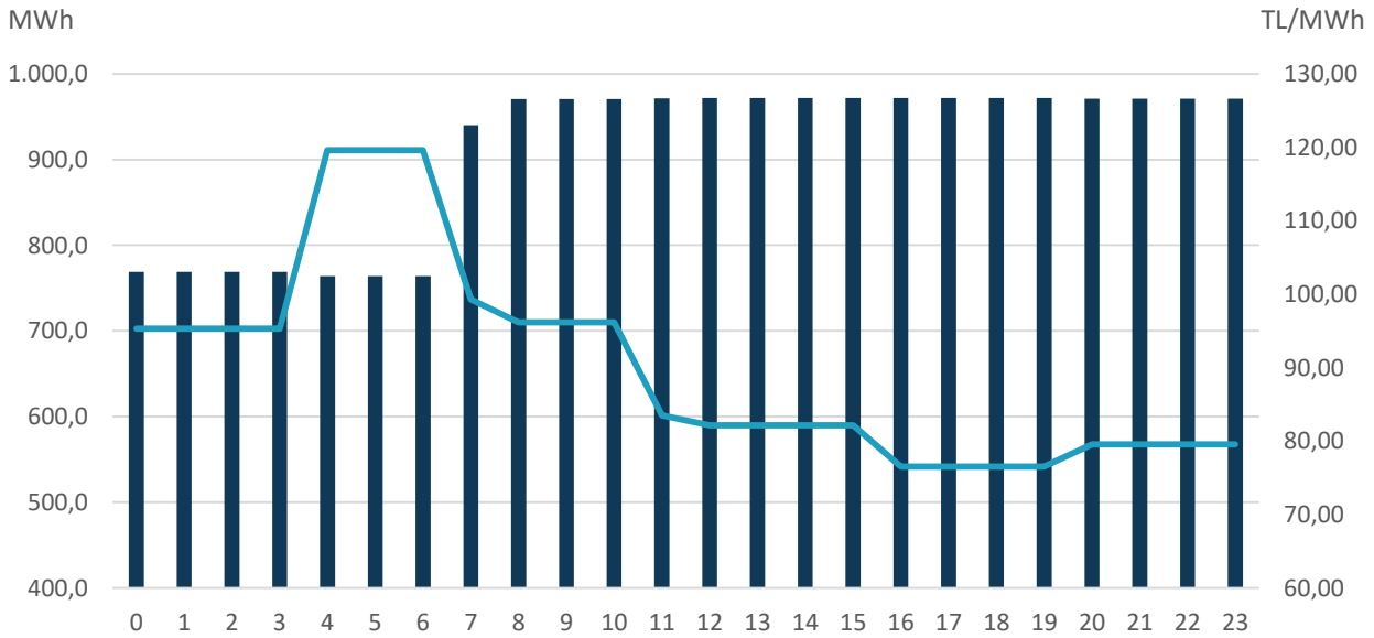
Grafik 43:Saati Ortalama SFK Rezerv Miktarı ve Ağırlıklı Ortalama Fiyatı
