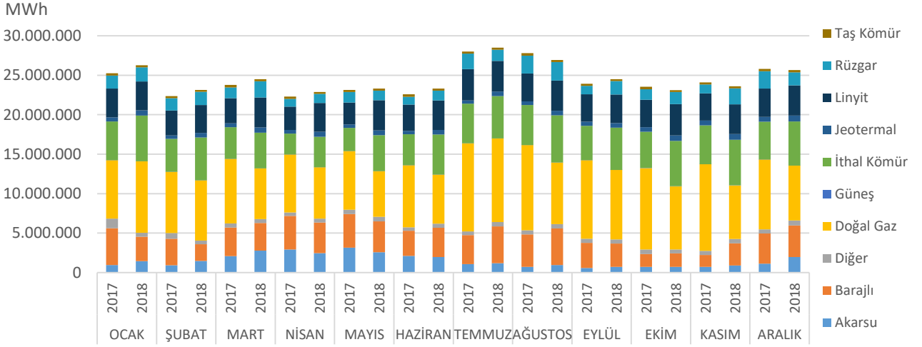
Grafik 67: 2017 - 2018 Yılları Kaynak Bazında Üretim Değerleri
