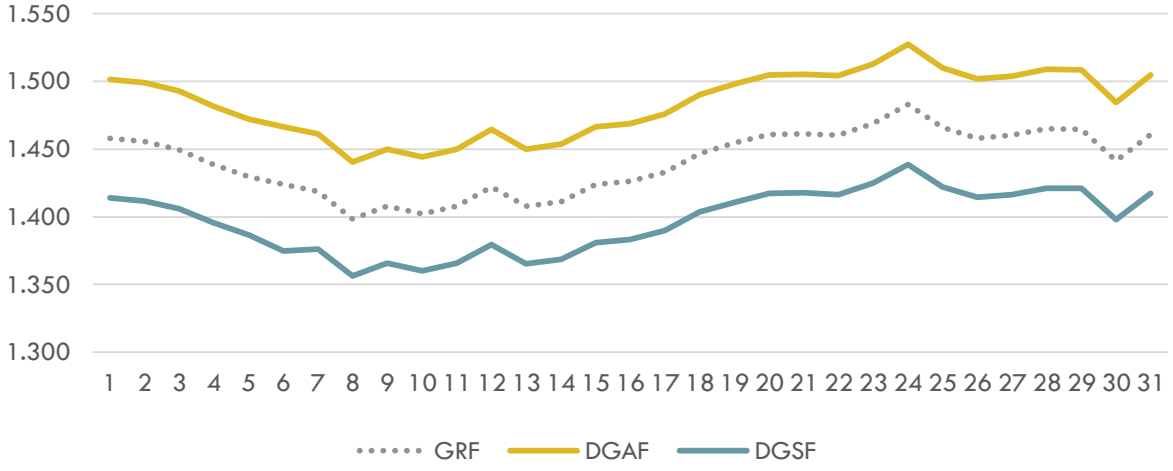
Mart 2020 GRF - DGAF – DGSF (TL/'000 Sm 3 )
