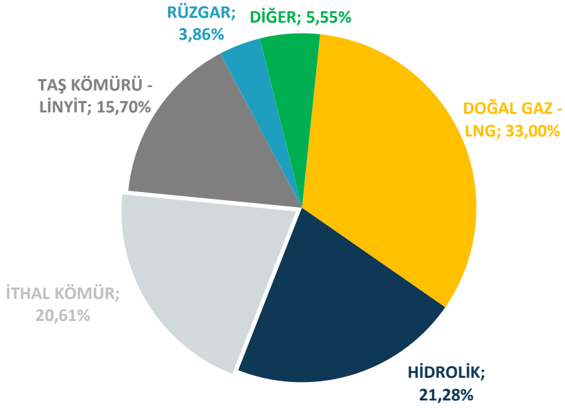
ELEKTRİK ÜRETİMİNDE KAYNAK DAĞILIM GRAFİĞİ (41. HAFTA)
