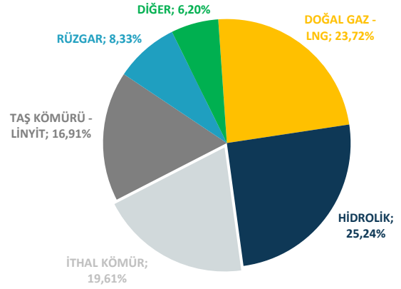
ELEKTRİK ÜRETİMİNDE KAYNAK DAĞILIM GRAFİĞİ (25. HAFTA)
