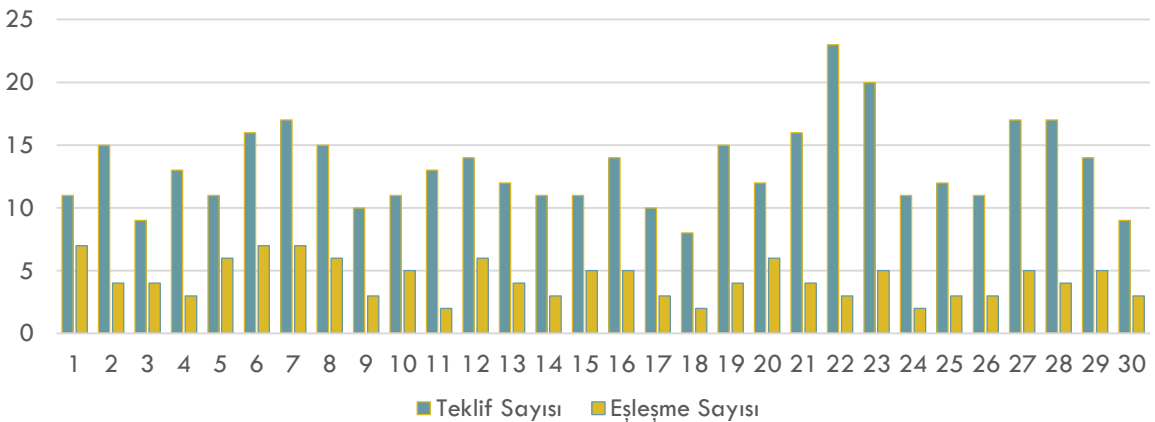
Haziran 2022 Doğal Gaz Piyasası Teklif ve Eşleşme Sayısı
