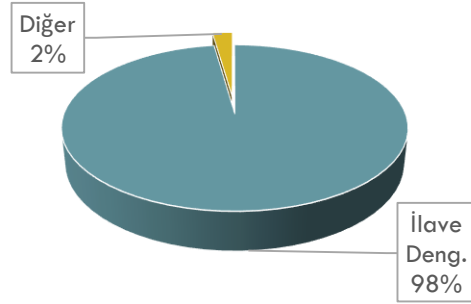
Haziran 2022 Dönemi İlave Dengeleyici Eşleşme Miktarı
