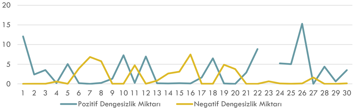
Haziran 2022 Dönemi Negatif ve Pozitif Dengesizlik Miktarı (mio.Sm 3 )
