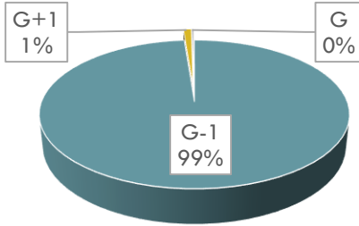
Haziran 2022 Dönemi Günlük Kontratların Seanslara Göre Eşleşme Miktarı
