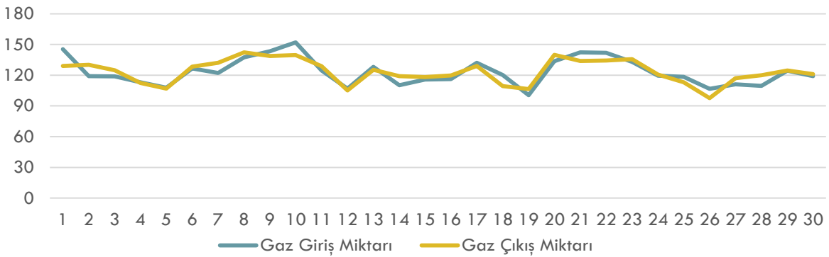
Haziran 2022 Gaz Giriş ve Çıkış Miktarı (mio.Sm 3 )
