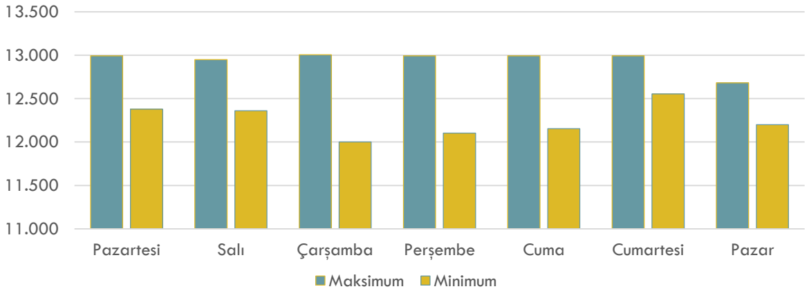
Haziran 2022 Doğal Gaz Piyasası Günlere Göre Maks. / Min. GRF (TL/'000 Sm 3 )
