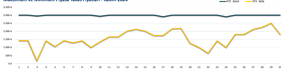
Maksimum ve Minimum Piyasa Takas Fiyatları - Kasım 2024
