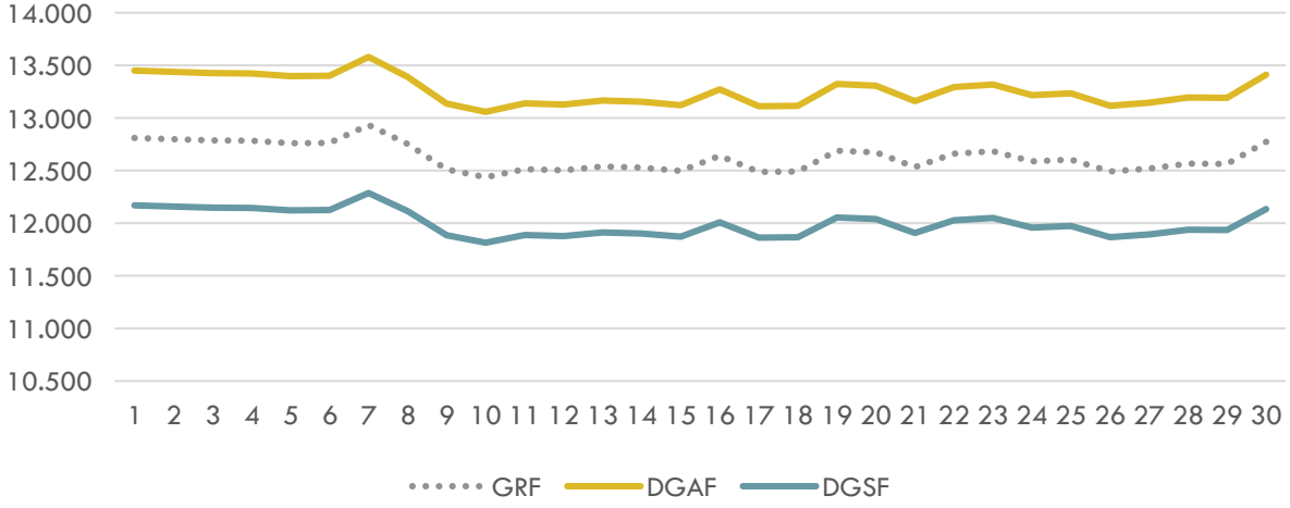
Nisan 2025 GRF - DGAF – DGSF (TL/'000 Sm 3 )
