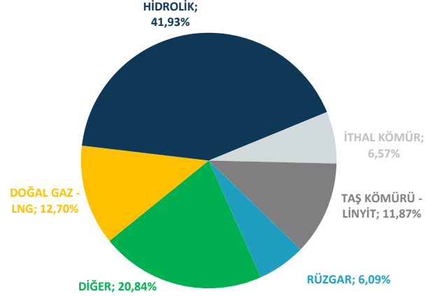
ELEKTRİK ÜRETİMİNDE KAYNAK DAĞILIM GRAFİĞİ (19. HAFTA)
